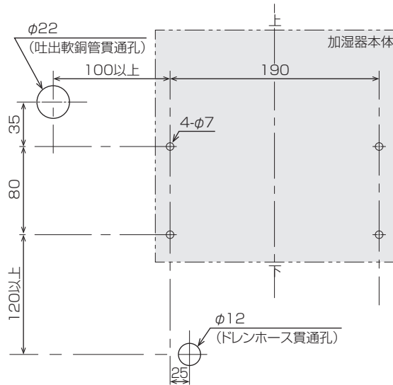
図3：加湿器本体取付孔寸法(全型番共通)
