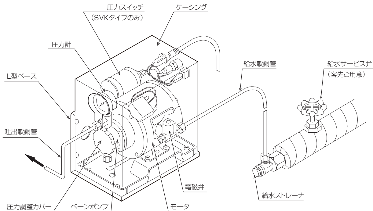
図 11：各部の名称
