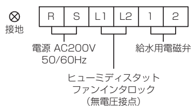
図-5 端子台接続図
