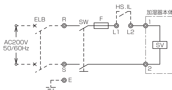
図-4 電気回路図
