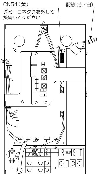
図 - 15 空調機制御ボックス内基板
