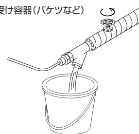
(図9) 給水ストレーナからフラッシングする場合
