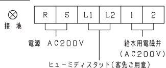
端子台接続図
