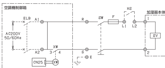
端子台接続図
