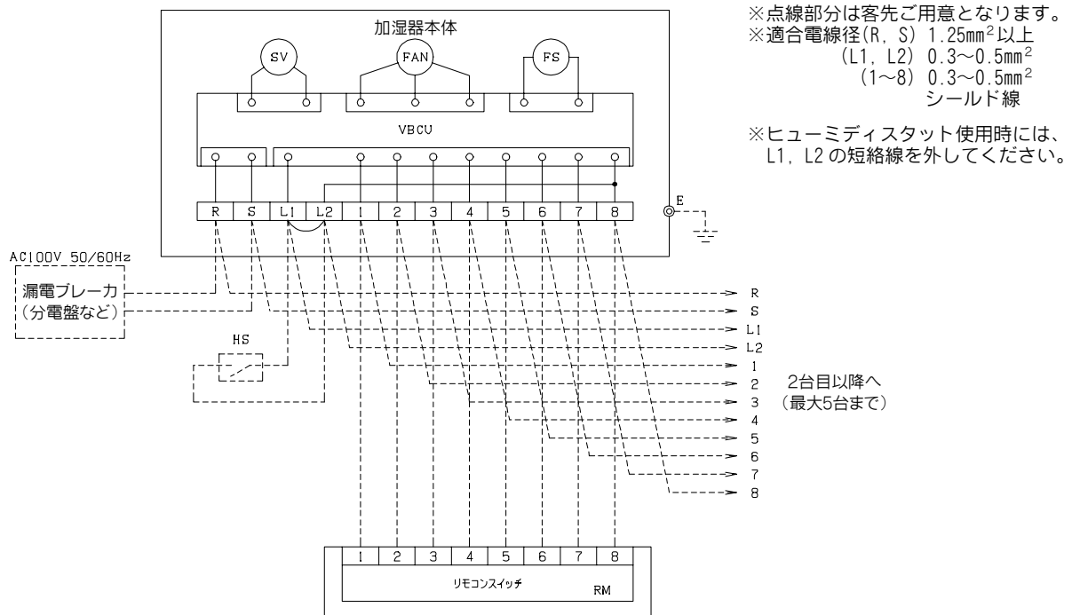
図-6 結線要領
