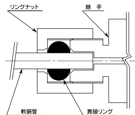
図-4 給水軟銅管の接続
