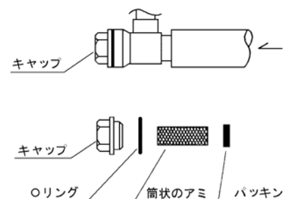
図-9 ストレーナ分解図
