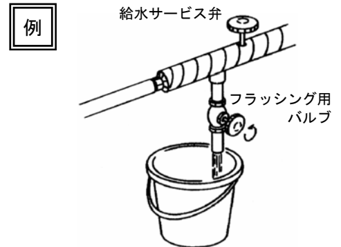
図-8 給水配管のフラッシング
