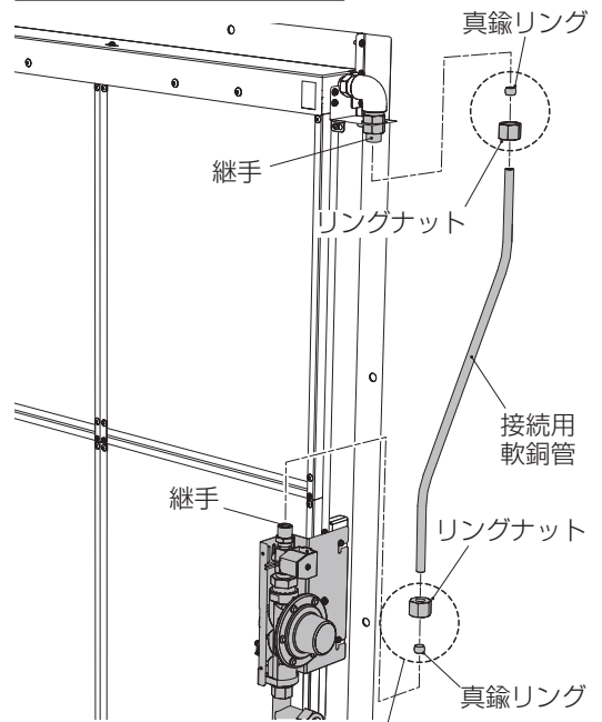
図-19：接続用軟銅管の接続
