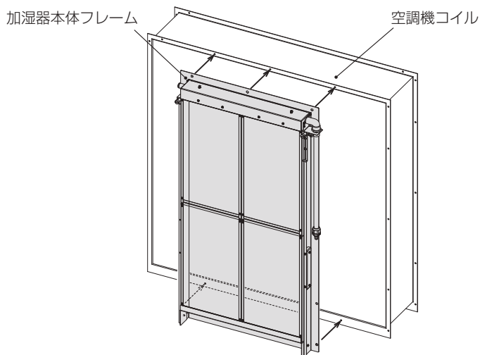
図-5：オープン方式の取付（縦固定）
