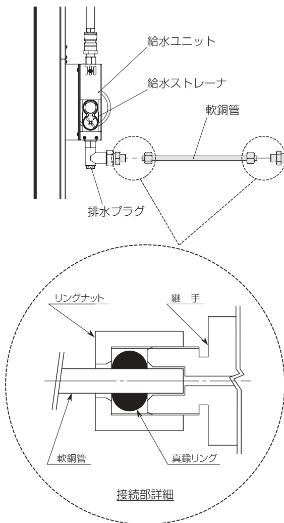
図-20：給水軟銅管の接続
