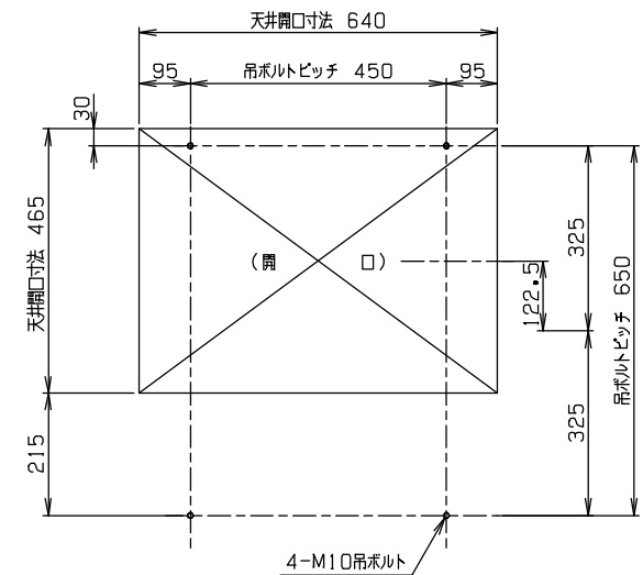
図-2 吊り込み寸法
