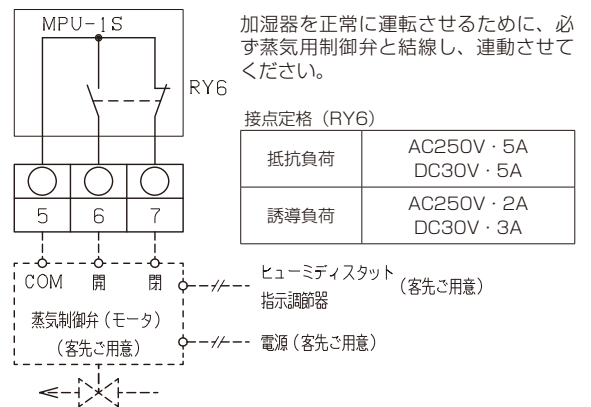
図-13 結線例
